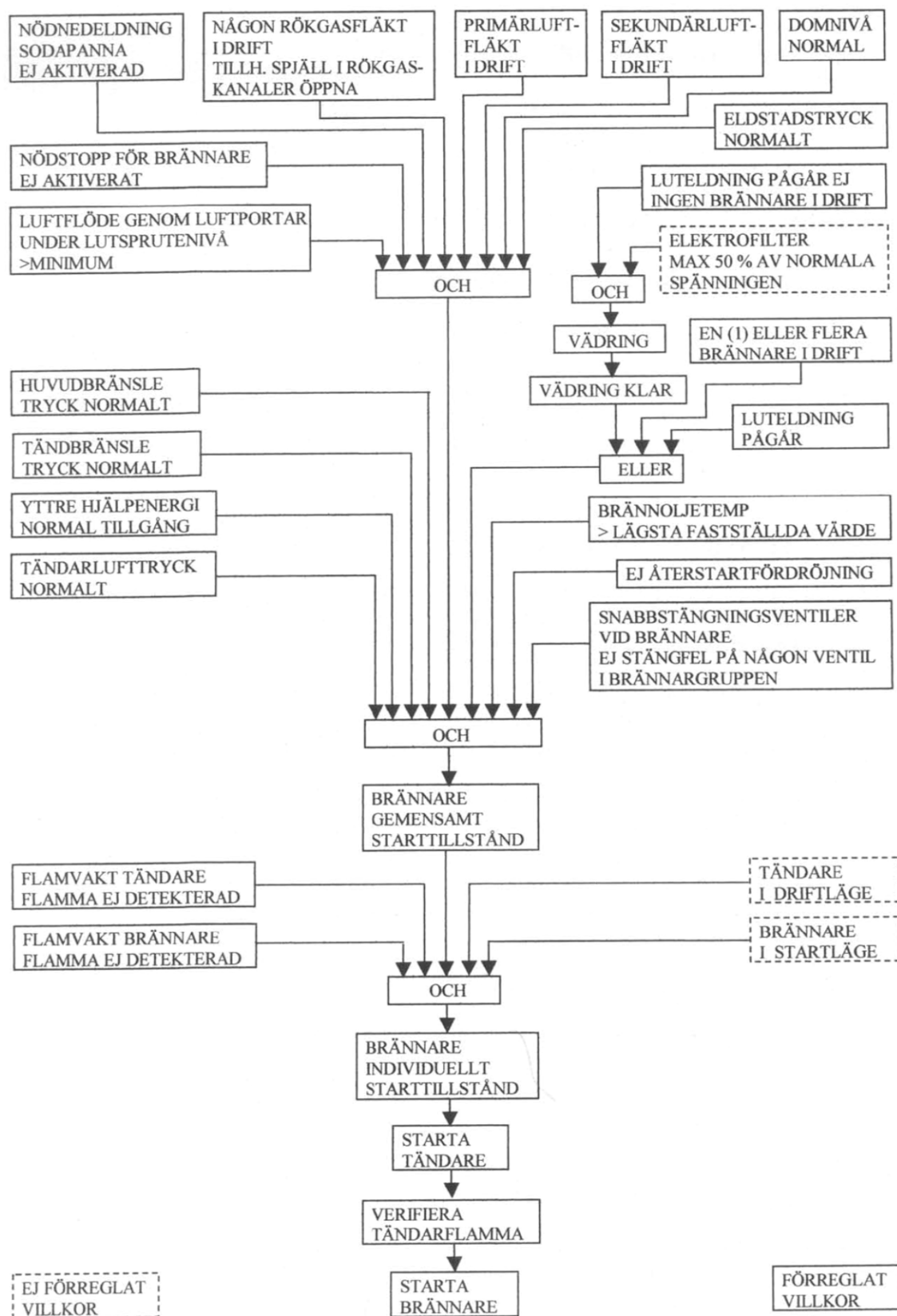
Figur 1, Exempel på startvillkor för oljeeldade startbrännare
